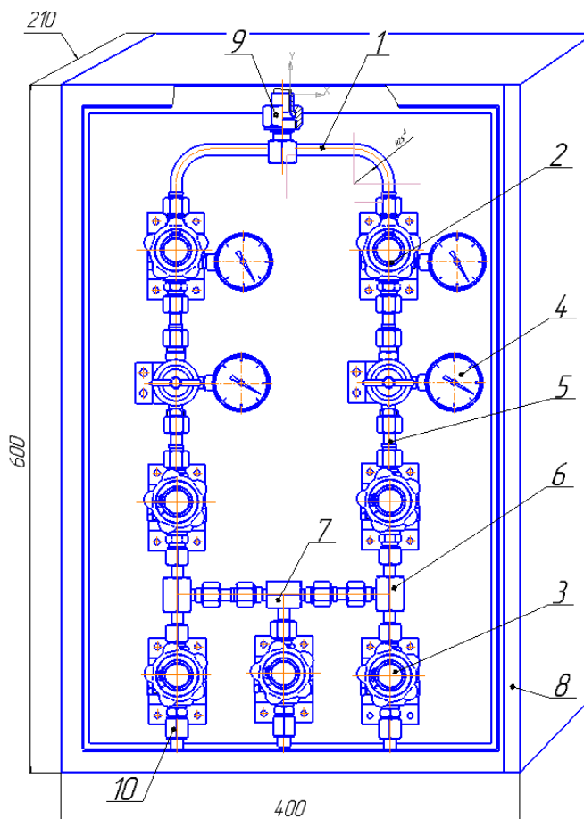
Рис. 1. Пост газопитания ПГКЗ-20-з
